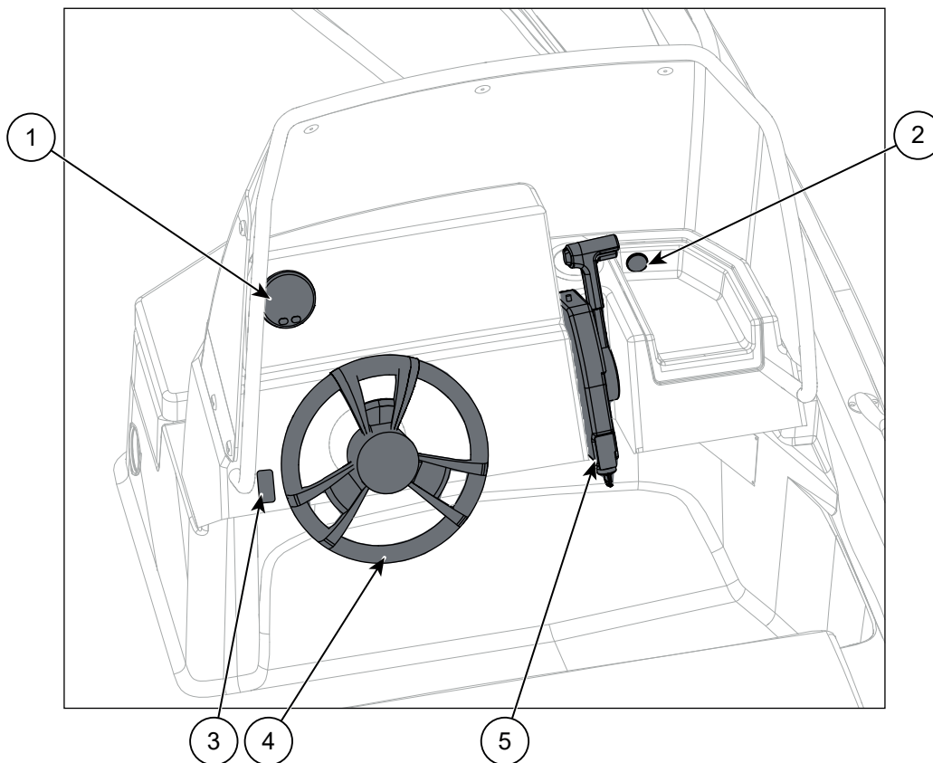
Figur 5.1 Yamarin 46 SC styrestasjonskontroller
