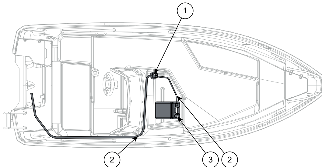
Figur 6.1 Yamarin 46 SC komponenter i drivstoffsystem
