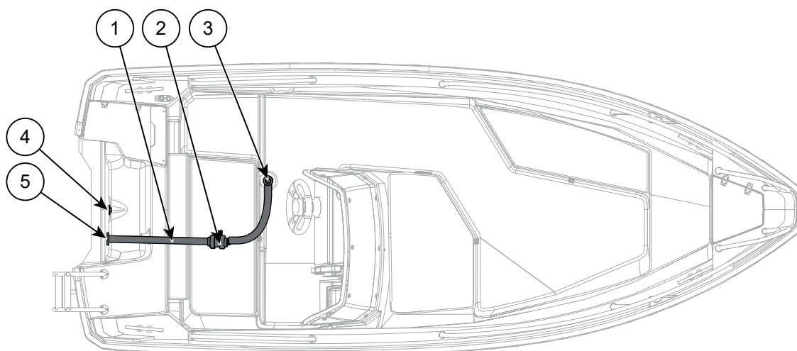
Figur 9.1 Yamarin 46 SC dreneringsutstyr
