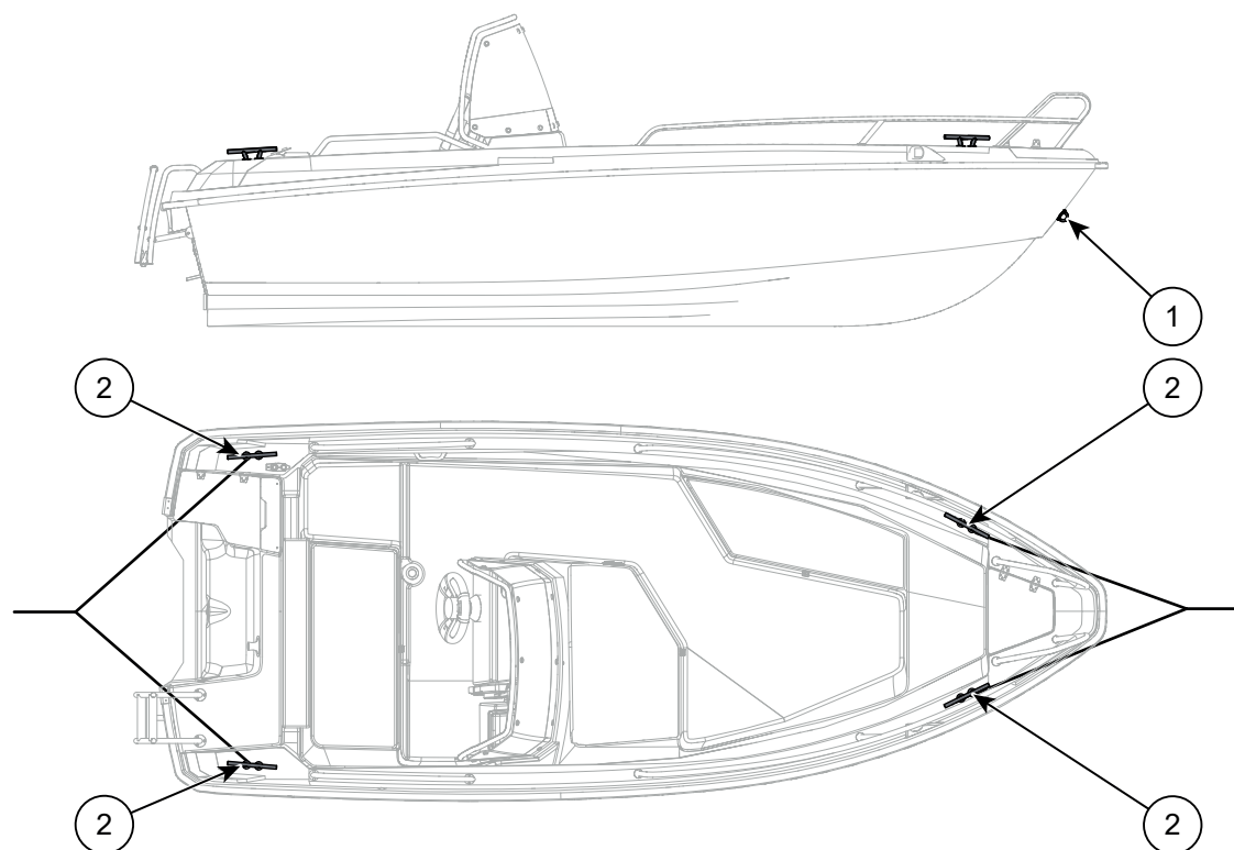
Figur 5.3 Yamarin 46 SC fortøynings- og slepepunkter
