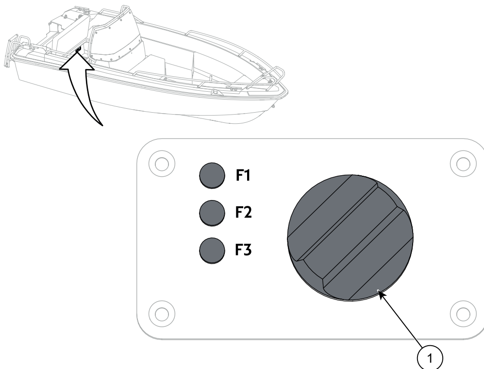
Figur 8.1 Yamarin 46 SC beskrivelse av brytere og sikringer
